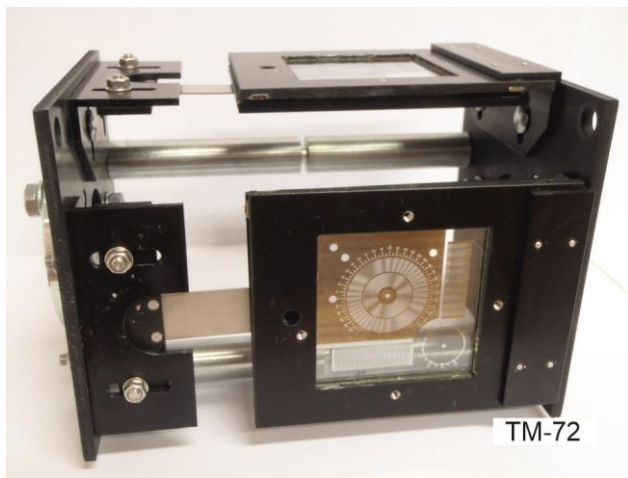
Extensometr TM72
